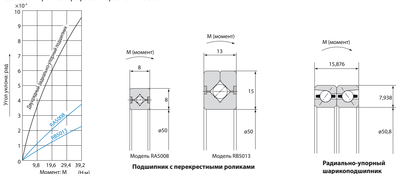
Диаграмма жёсткости моментов
