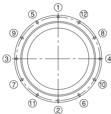
Рис. 1 Порядок затяжки
