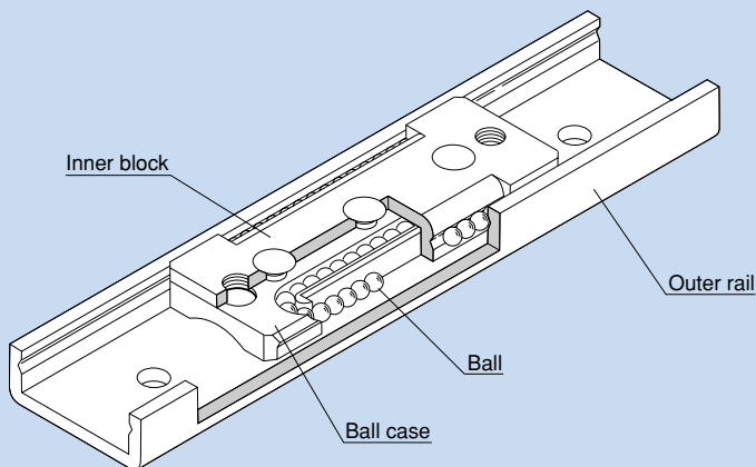
Fig. 1 Structure of Precision Linear Pack Model ER
